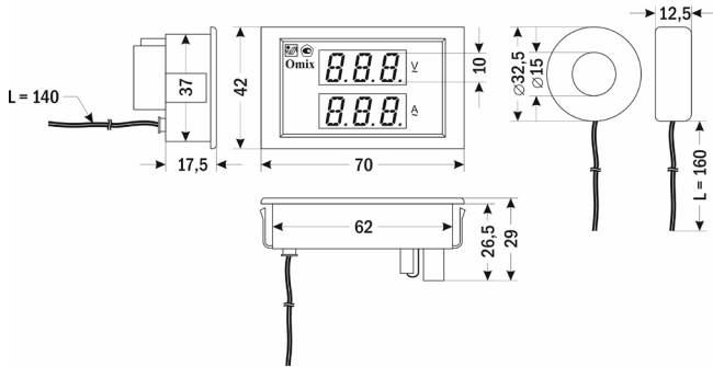
Рис. 3 – Размеры прибора
